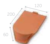
Cuña para caballete
