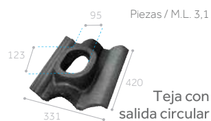
Teja de ventilación
