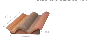
Teja de alero
