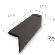
Remate lateral perfil ancho izqdo
