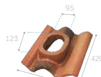
Teja de ventilación
